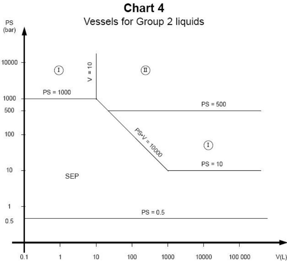
Dijagram 1: Klasa posude (2014/68/EU)
